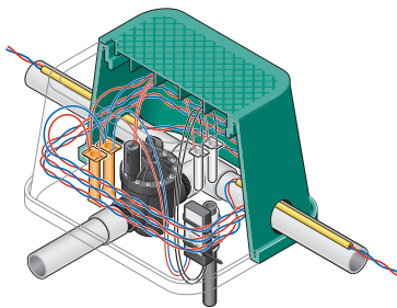
Decoder im Ventilkasten
